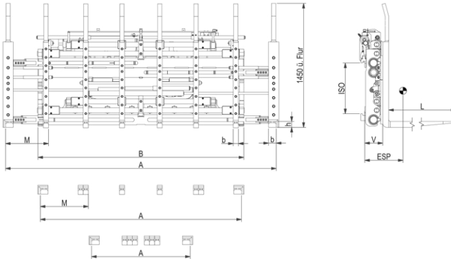
Vierfachpalettengabel 2-3-4 Paletten
