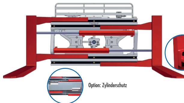
angeschraubte Gabelzinken
