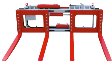
Bild zeigt Typ DST mit Sonderausstattung Gabelzinken angeschraubt
